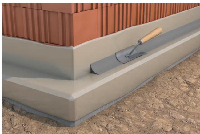
1.4 Hohlkehle setzen ( INTRASIT® RZ1 55HSP oder INTRASIT® FSM Winter 56Z )
